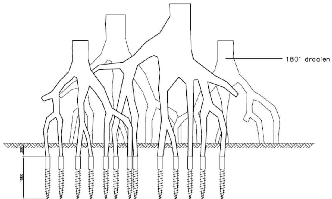
Voorraanzicht (schaal 1:50)
